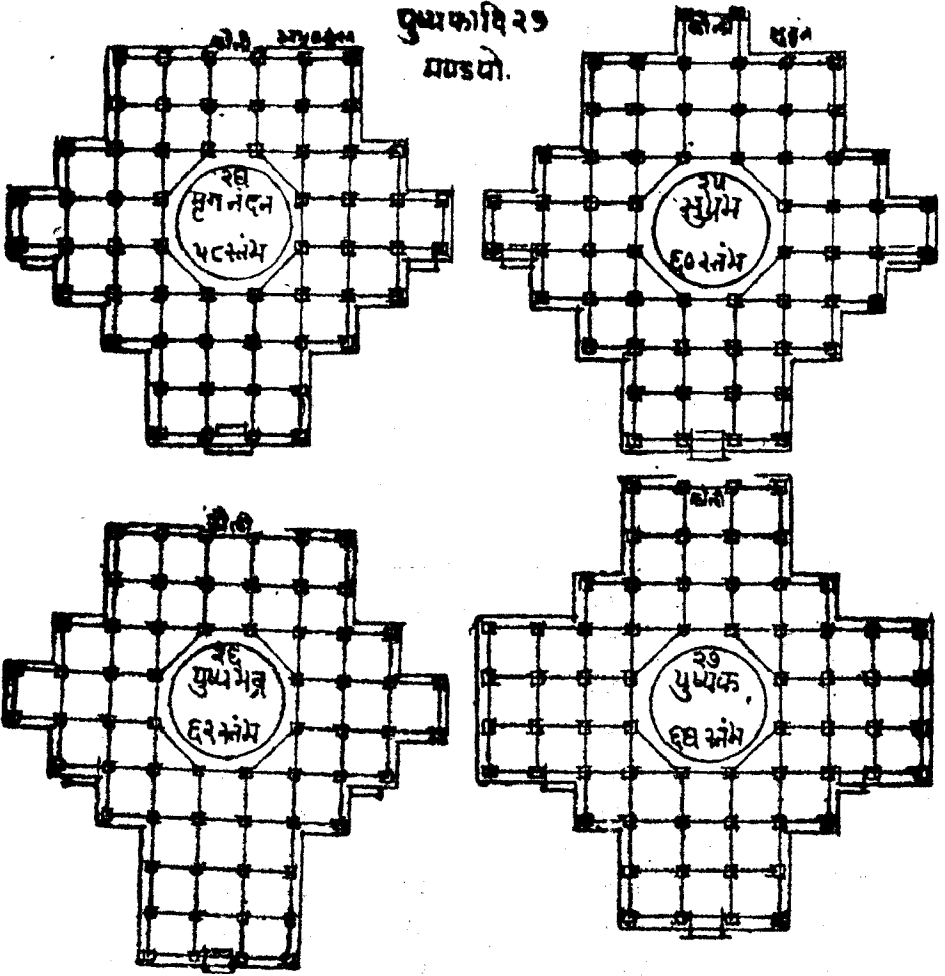
पुष्पकादि २७ मंडपोमांता २४-२७ मंडपोना आलेखनो
