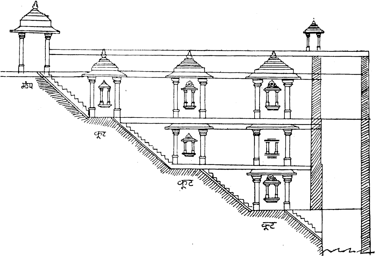
વાવનું સેકશન
