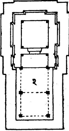
६ स्तंभनी
