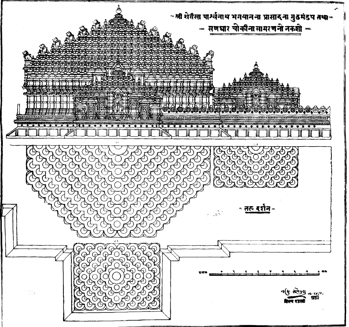
श्रीपार्थिनाथ भगवानना देरासरना गूढ मंडपना नकशो. शेरीसा, ( उत्तर गुजरात ).
